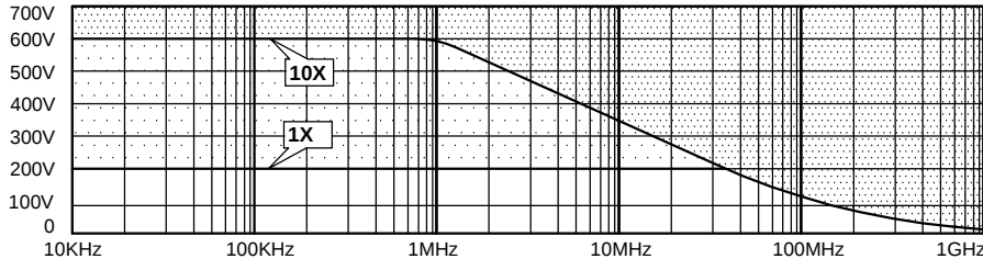
电压-频率特性图 (VDC+Peak AC)
